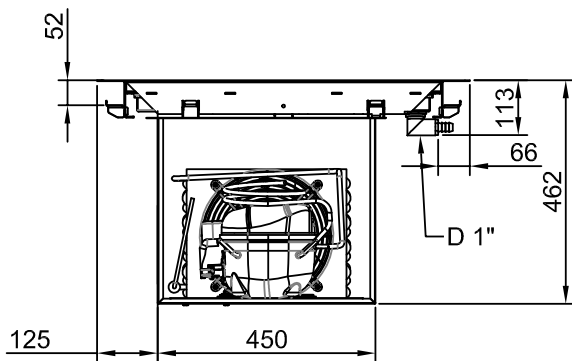
Zij aanzicht
