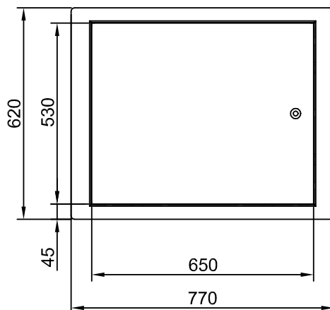
Boven aanzicht
